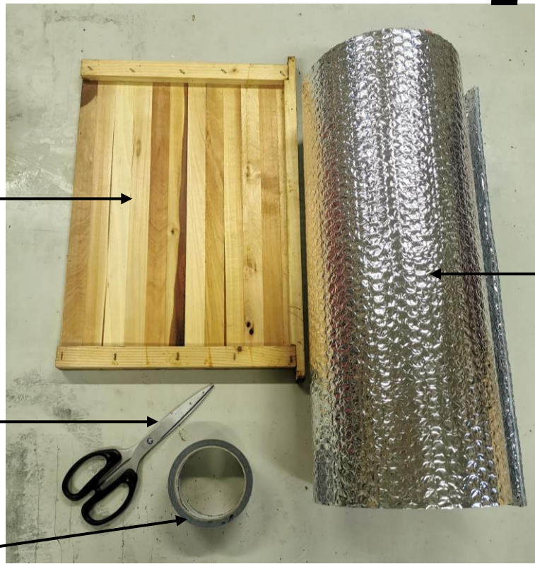
Matériel nécessaire pour fabriquer une partition isolante Jade Laumain
